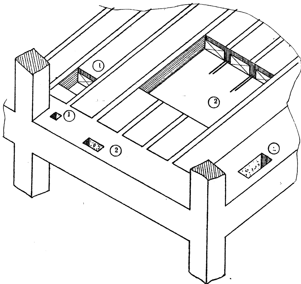
Fig. 3-7.. ① Perì che non richiedono revisione delle strutture portanti ② Perì che richiedono rafforzamenti delle strutture (solai e travi) interessate.
