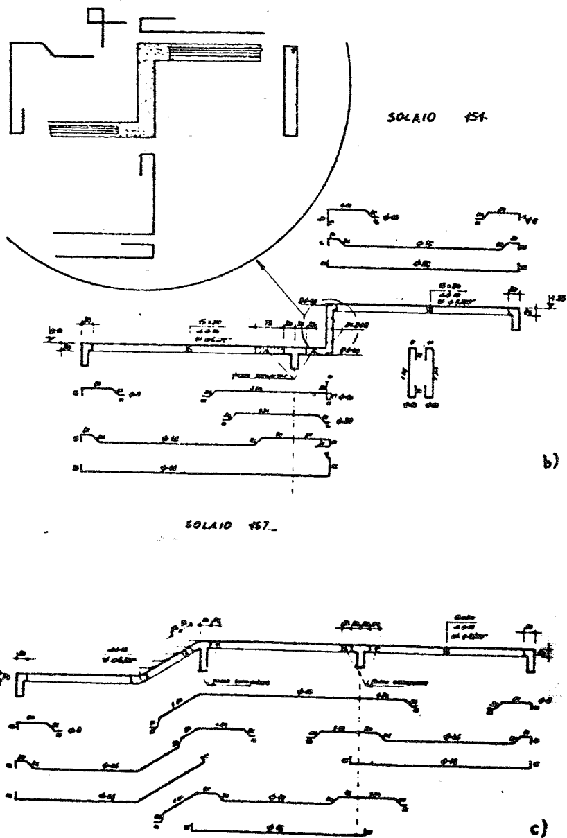
Fig. 3 17 b) c) b) Armature di un solaio ad asse spezzato della carpenteria di fig. 3 17a) (in alto altre possibili disposizioni delle armature). c) Nella prima campata il solaio presenta un tratto ad asse inclinato.
