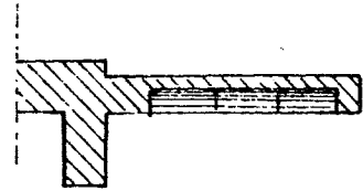
sbalzo con soletta alleggerita con blocchi in laterizio.
